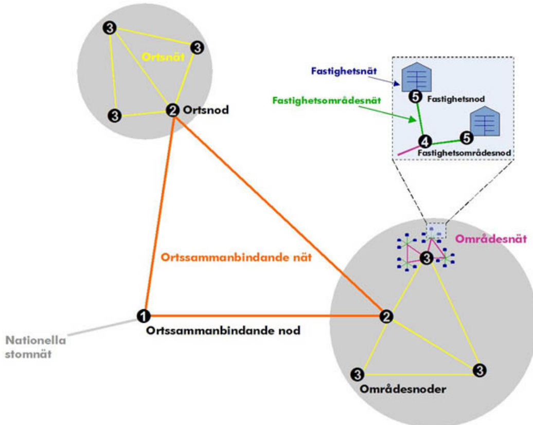
Principbild på nätstruktur
